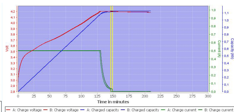
Charakterystyka ładowania ogniwa ICR18650-260PCM
