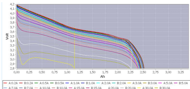
Charakterystyka rozładowania ogniwa ICR18650-260PCM
